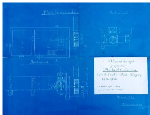
Planul morii, întocmit în anul 1926
